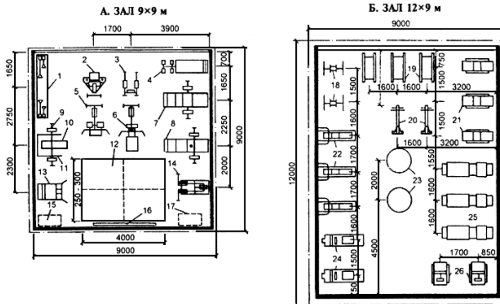
ЭКСПЛИКАЦИЯ ДЛЯ А И Б
