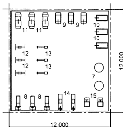
В. ЗАЛ 12×12 м ДЛЯ ЗАНЯТИЙ НА ТРЕНАЖЕРАХ
