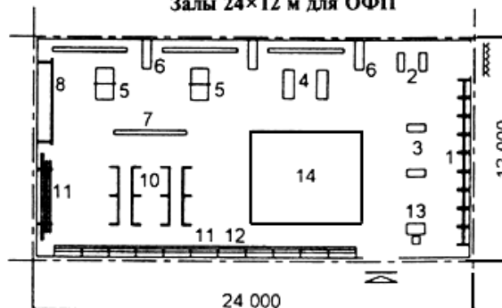
Залы 24×12 м для ОФП
