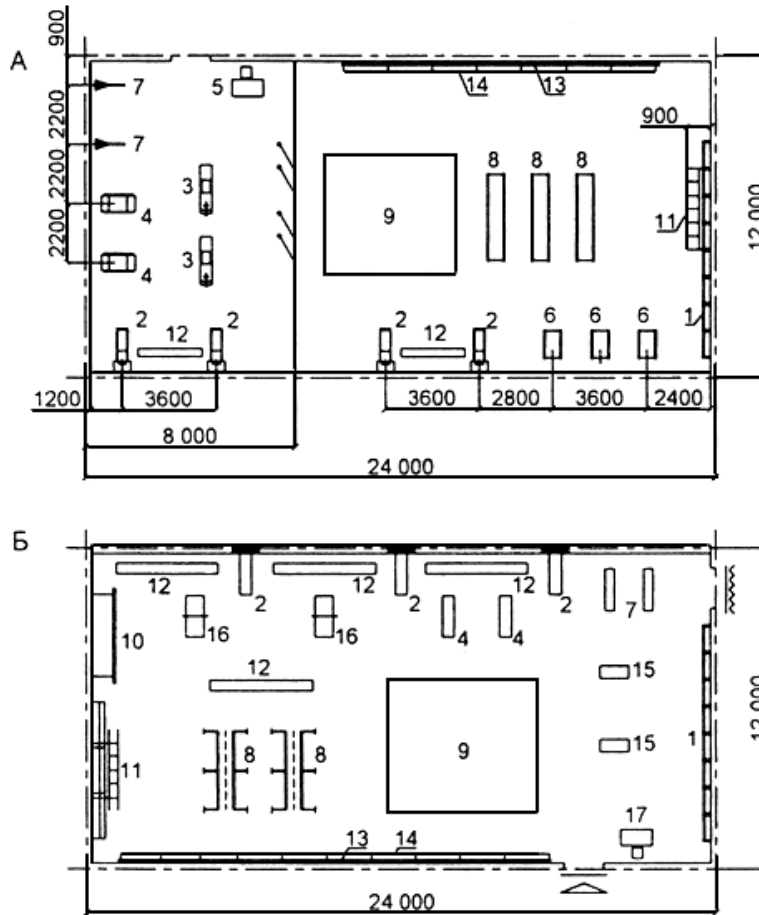
ВАРИАНТЫ ОБОРУДОВАНИЯ ЗАЛА 24×12 м
