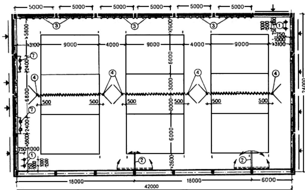
ЗАЛ ДЛЯ ВОЛЕЙБОЛА
