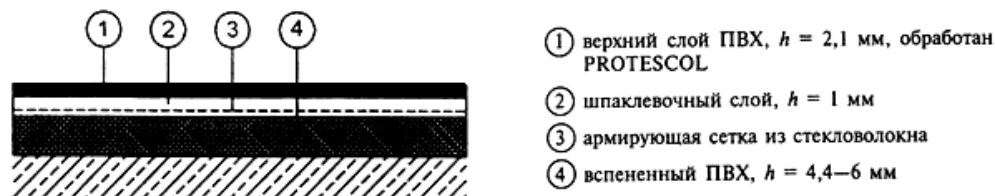
Схема 4. Пол с синтетическим покрытием рулонного типа
