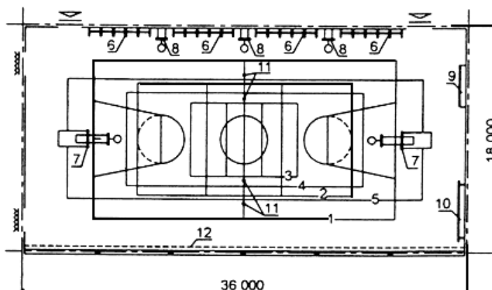
СХЕМА РЕШЕНИЙ ЗАЛОВ ДЛЯ ОФП И ТРЕНИРОВОК
