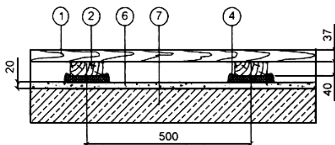
Схема 2. Пол по двойным лагам
