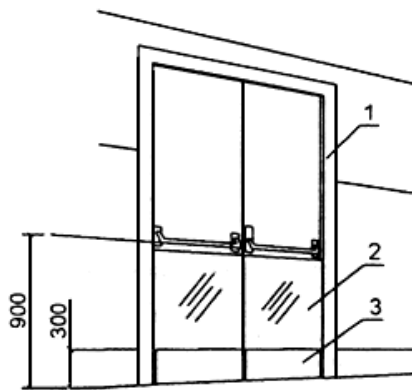
Схема входной двери в зал
