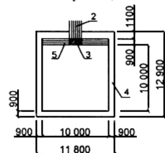
Зал с уменьшенной полосой ориентации
