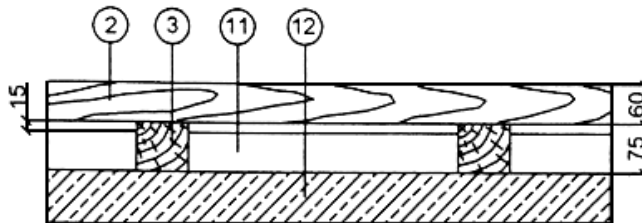
Схема 4. Брусчатый пол по лагам на перекрытии
