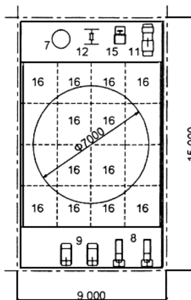
Б. ЗАЛ 15×9 м ДЛЯ ГРУППОВЫХ ЗАНЯТИЙ ЭЛЕМЕНТАМИ БОРЬБЫ
