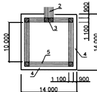
Зал нормальных размеров
