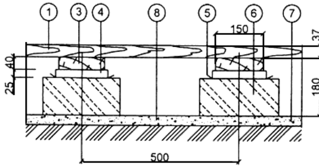
Схема 2. Дощатый пол по лагам на перекрытии
