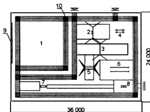
ЗАЛ 24×36 м ДЛЯ СПОРТИВНОЙ ГИМНАСТИКИ
