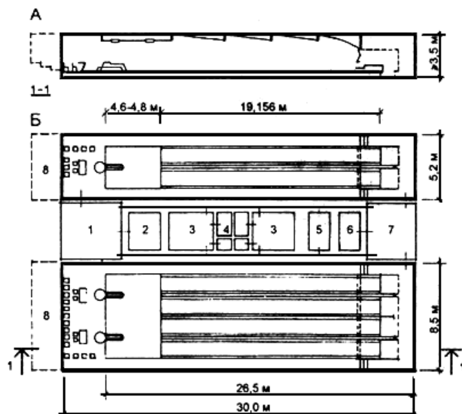
Планировочная схема кегельбана
