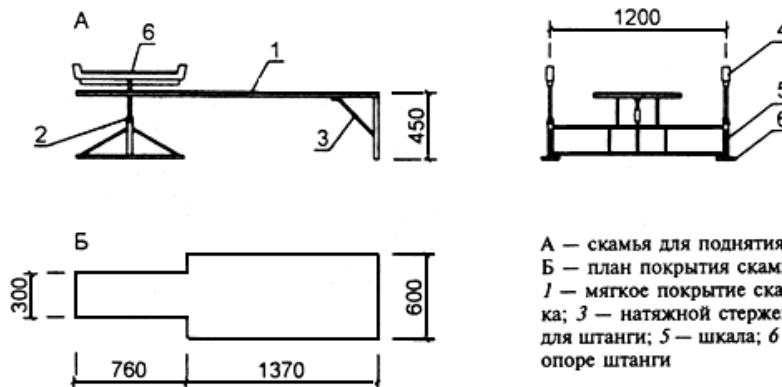
Скамья для занятий тяжелой атлетикой
