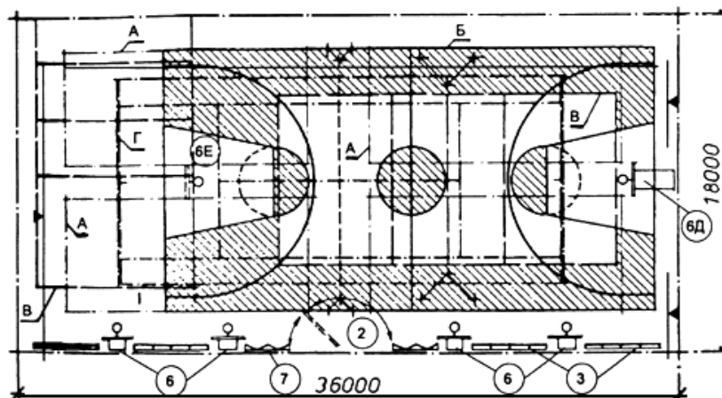
Б. Зал 36×18 м для: бадминтона (А), баскетбола (Б), волейбола (В), тенниса (Г)
