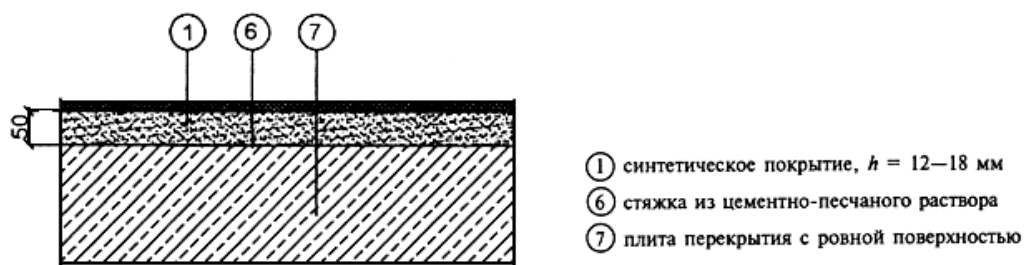
Схема 2. Пол по перекрытию
