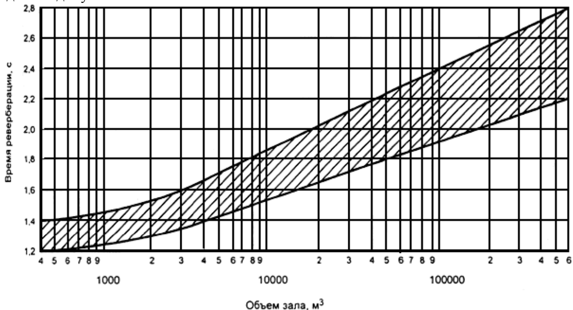
Рисунок 7.1 - График времени реверберации
