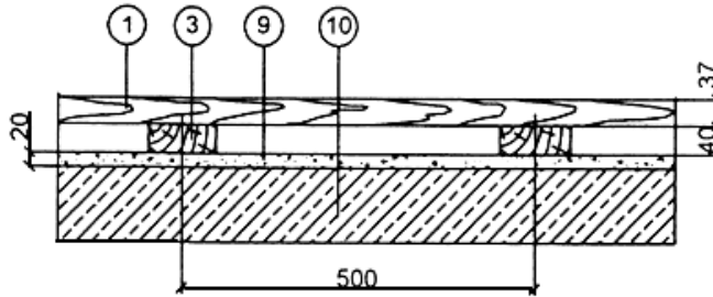
Схема 3. Брусчатый пол по лагам на грунте
