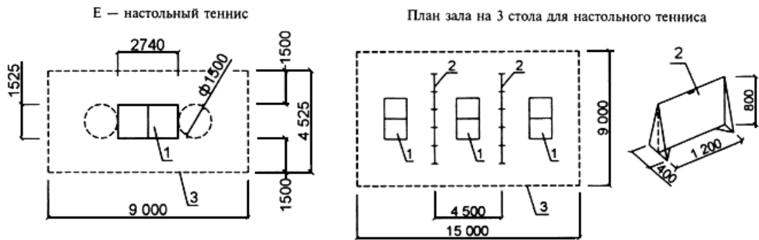
1 — стол для игры 2 — передвижные барьеры 3 — граница зоны безопасности
