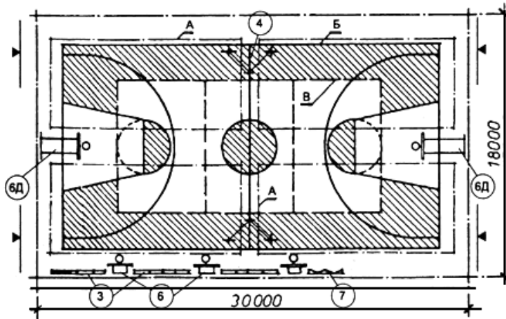
А. Зал 30×18 м для: бадминтона (А), баскетбола (Б), волейбола (В)
