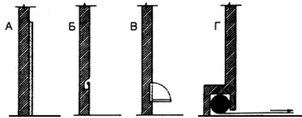
Особенности решения стен спортивных залов
