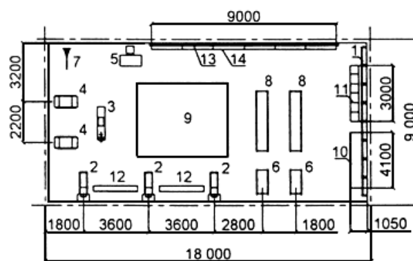
ОБОРУДОВАНИЕ ЗАЛА 18×9 м
