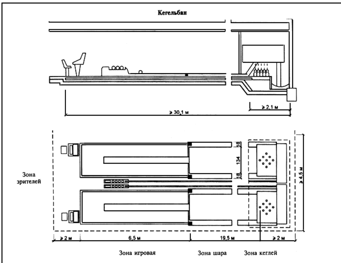
Планировочная схема кегельбана
