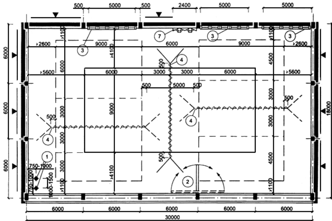
ЗАЛ РАЗМЕРОМ 30×18 м
