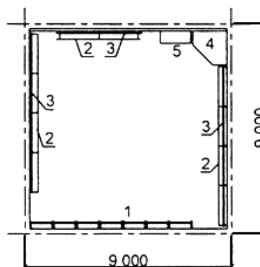
Г. ЗАЛ 9×9 м ДЛЯ ГРУППОВЫХ ЗАНЯТИЙ ПО РИТМИЧЕСКОЙ ГИМНАСТИКЕ, ХОРЕОГРАФИИ И ЖЕНСКОЙ ОЗДОРОВИТЕЛЬНОЙ ГИМНАСТИКЕ
