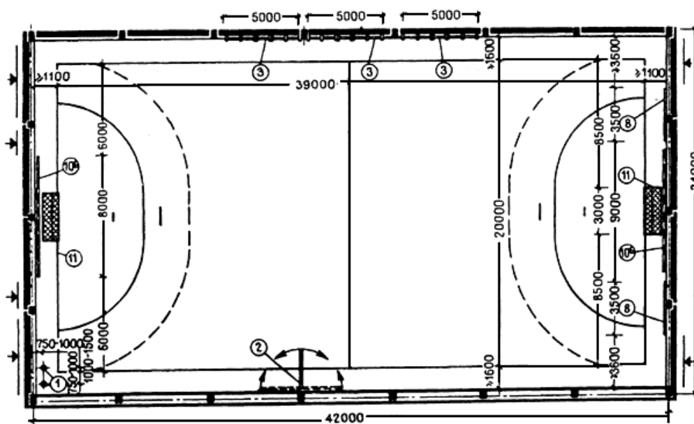
ЗАЛ ДЛЯ ГАНДБОЛА
