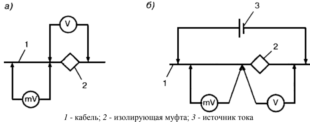
Рисунок 6 - Схема контроля состояния изолирующих муфт на кабелях приближенно без источника тока (а) и с источником тока (б)
