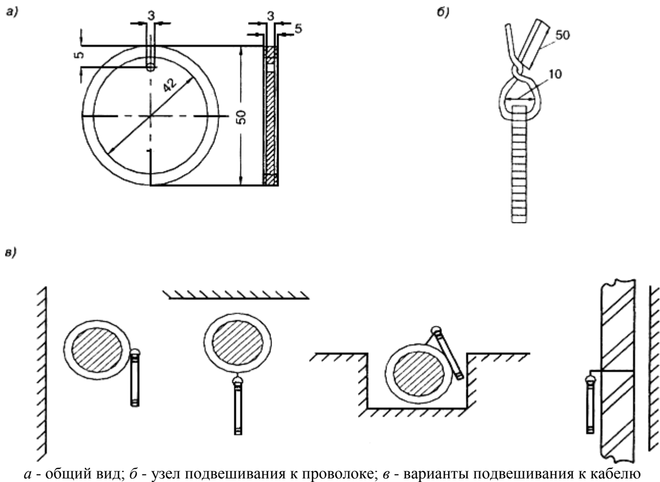
Рисунок 1 - Маркировочная бирка
