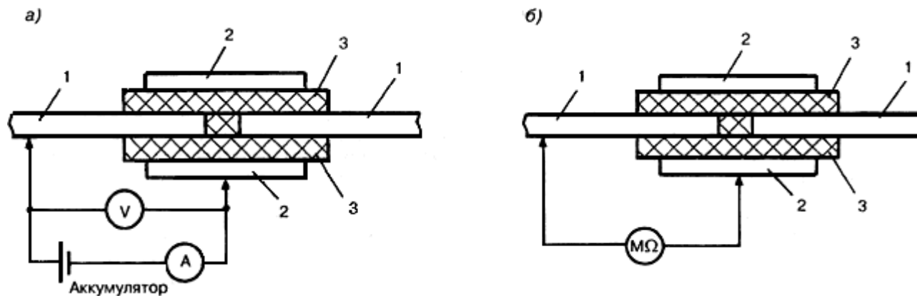
Рисунок 5 - Схема измерения сопротивления изоляции стыка ходового рельса
