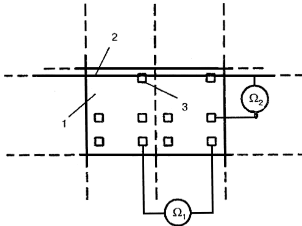
1 - блок; 2 - шина заземления; 3 - закладные детали
