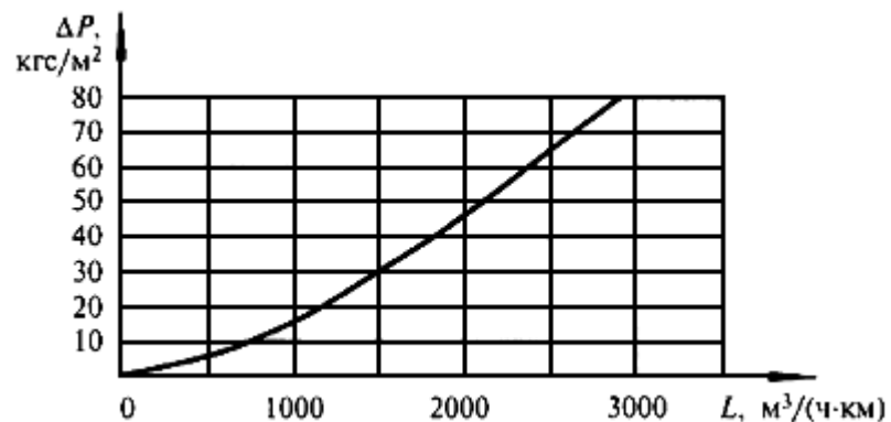
Рисунок 1 - График нормируемой утечки воздуха в испытываемом отсеке
