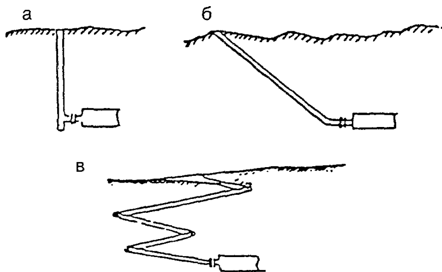
а - вертикальный ствол; б - наклонный ствол; в - наклонный спиральный ствол
