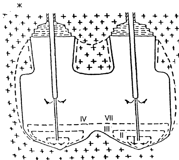
Рисунок 7. Технологические схемы сооружения выработок-емкостей бесшахтных резервуаров в каменной соли I - VII ступени сооружения выработок-емкостей
