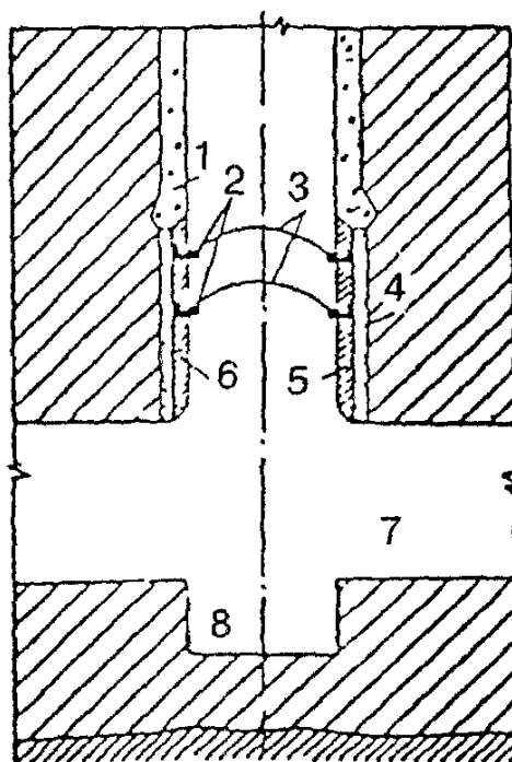
Рисунок 11. Двойная металлическая перемычка, расположенная в верхней части ствола
