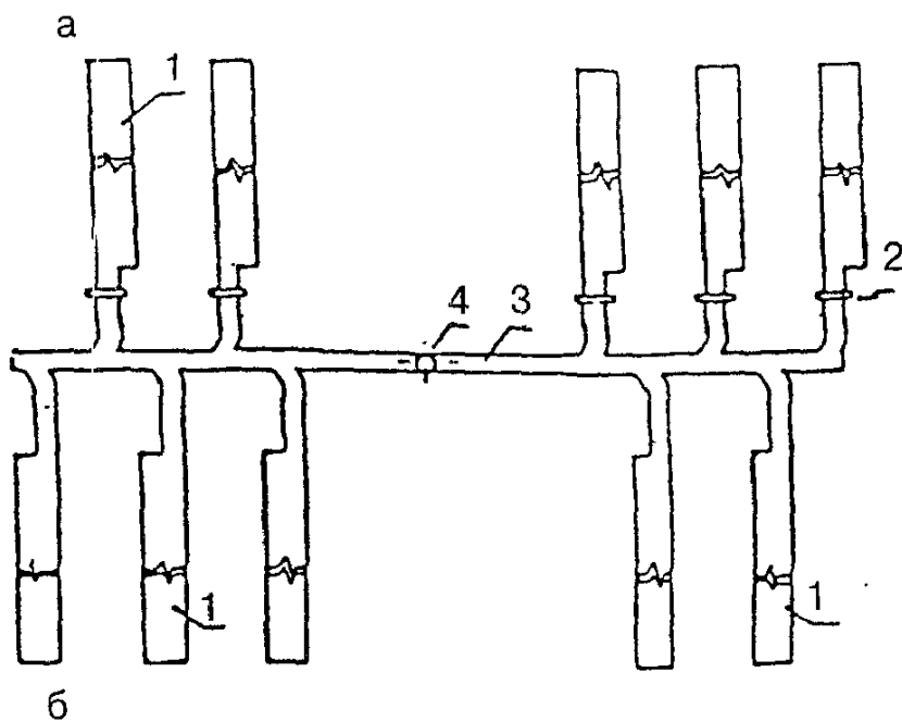
1 - выработка-емкость; 2 - герметичная перемычка; 3 - коллекторная выработка; 4 - ствол
