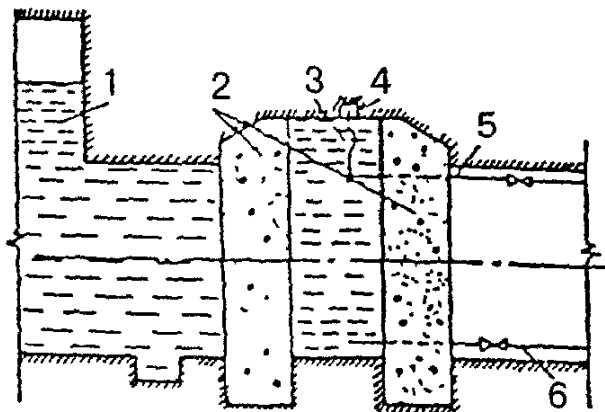
Рисунок 8. Бетонная перегородка с контурным гидрозатвором
