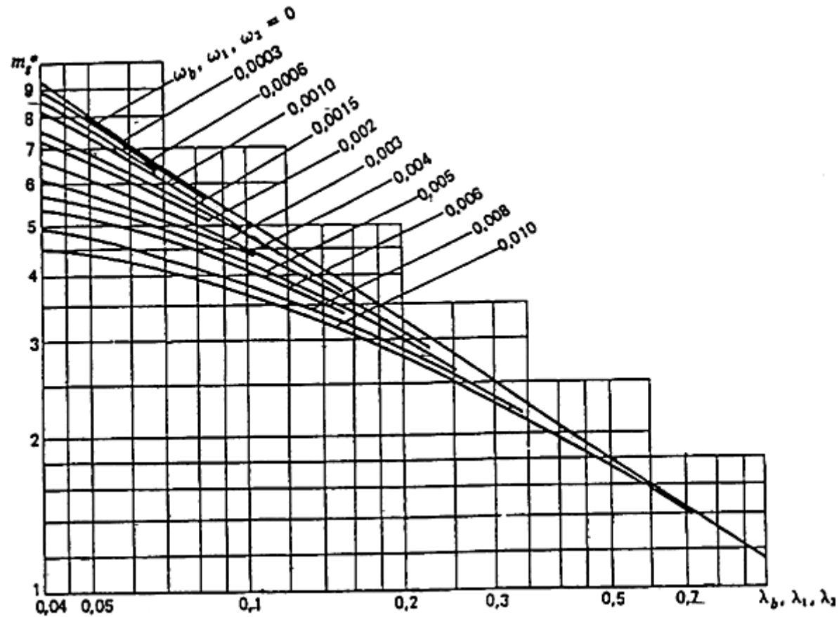
Рис.2. График для определения значений коэффициента m_s^*
