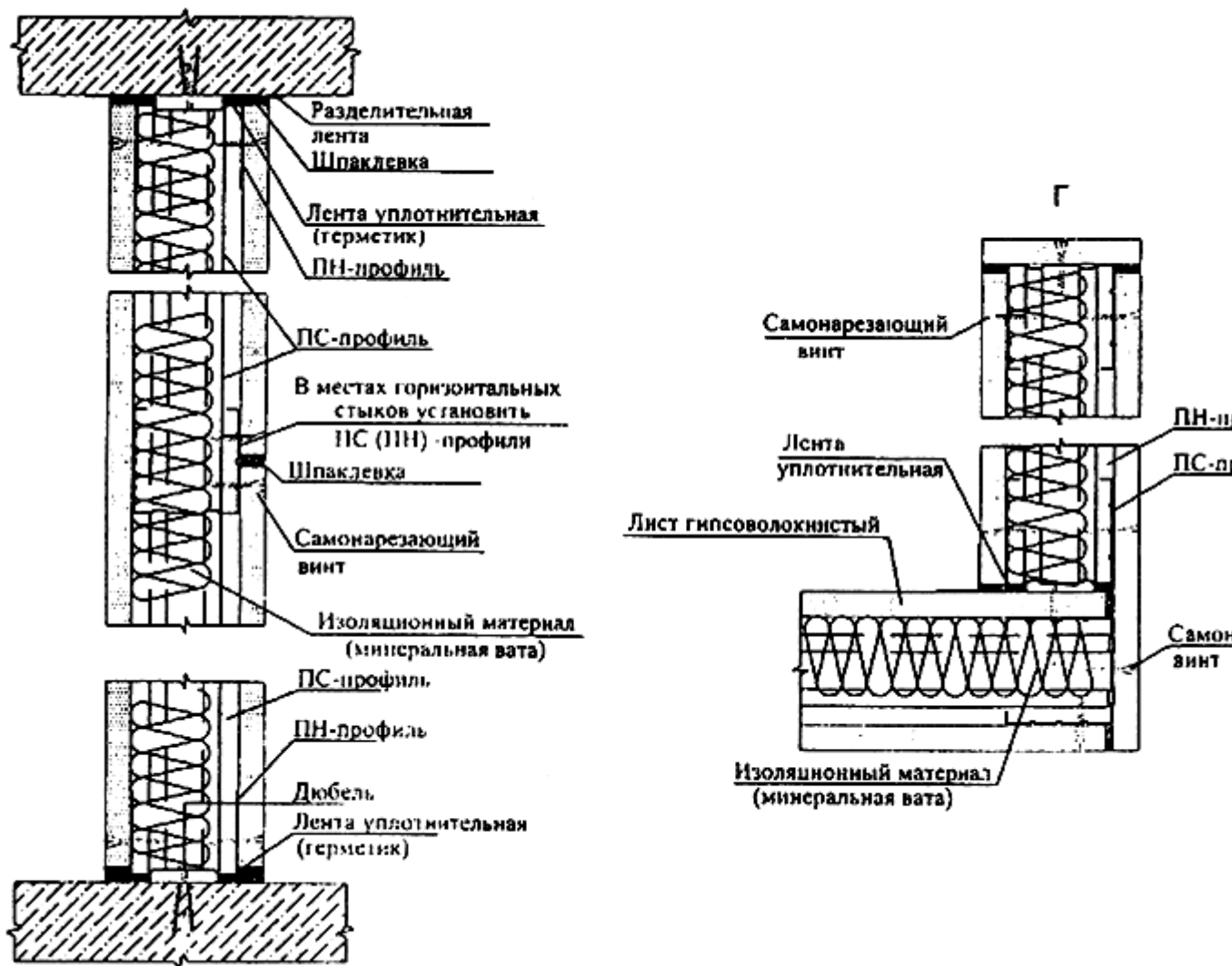
Рисунок 2 - Горизонтальный и вертикальный разрезы, узлы примыканий, внутренние и внешние углы перегородки с одинарной обшивкой гипсоволокнистыми листами на одинарном металлическом каркасе
