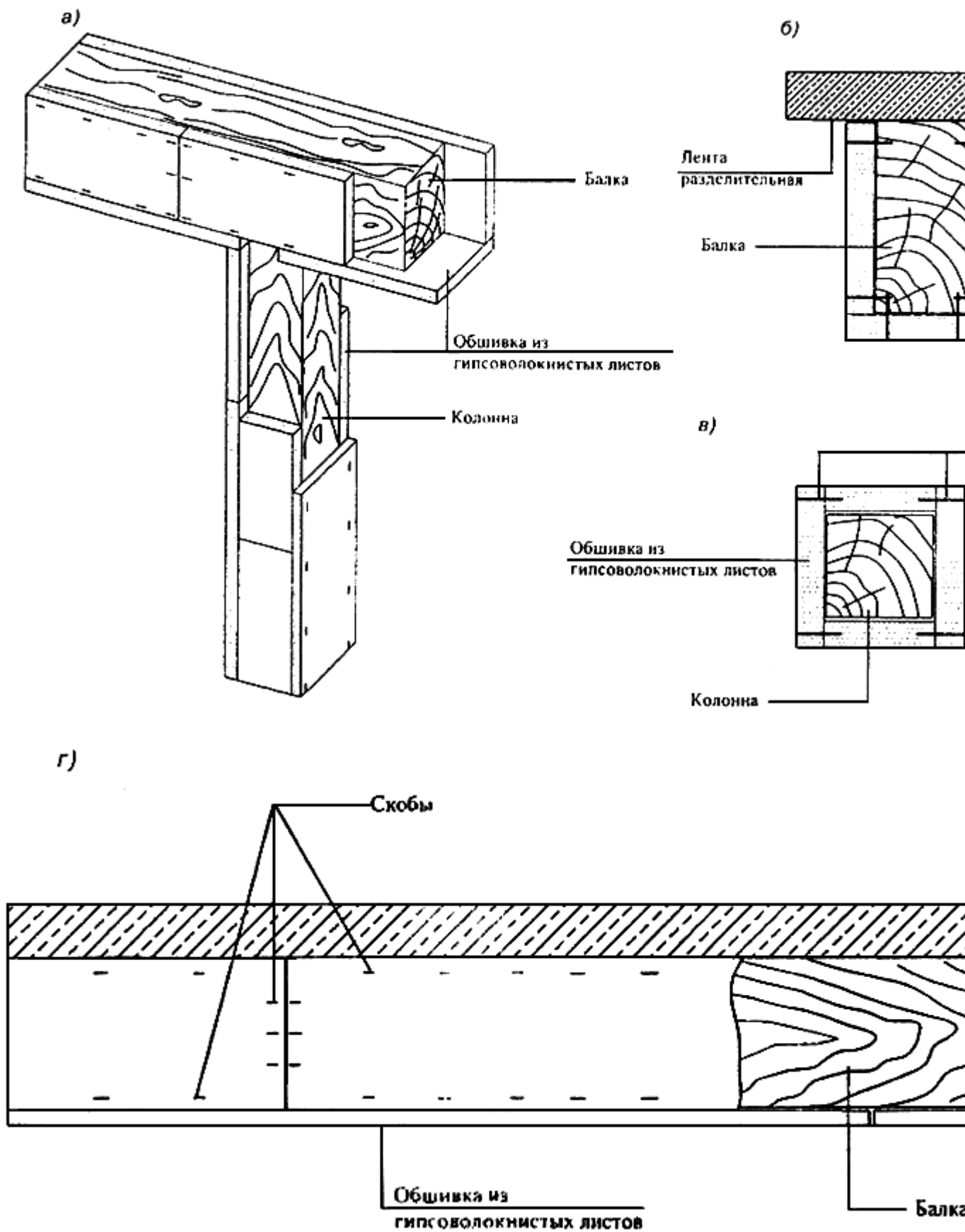
Рисунок 16 - Общий вид (а), конструктивное решение огнезащиты деревянной балки (б, г) и колонны (в)
