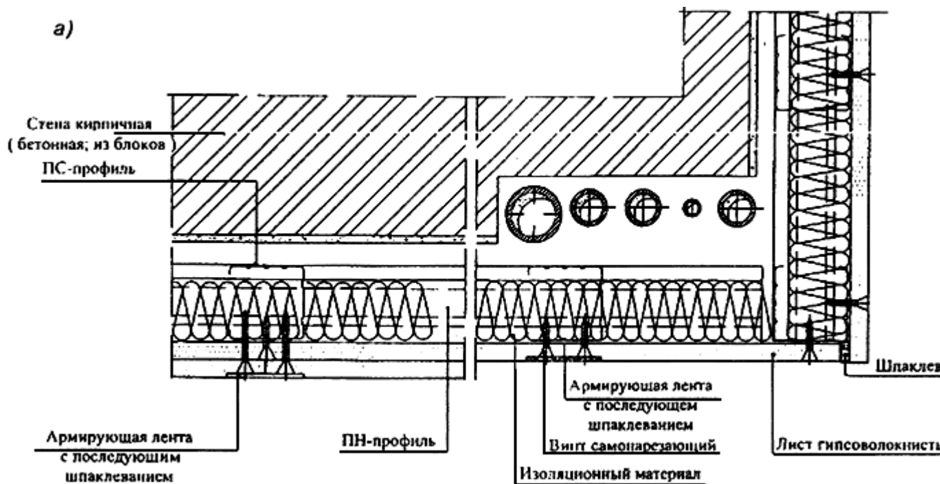
Рисунок 10 - Конструктивное решение оформления трубопроводов, размещенных вдоль капитальной стены (а), перегородки (б)
