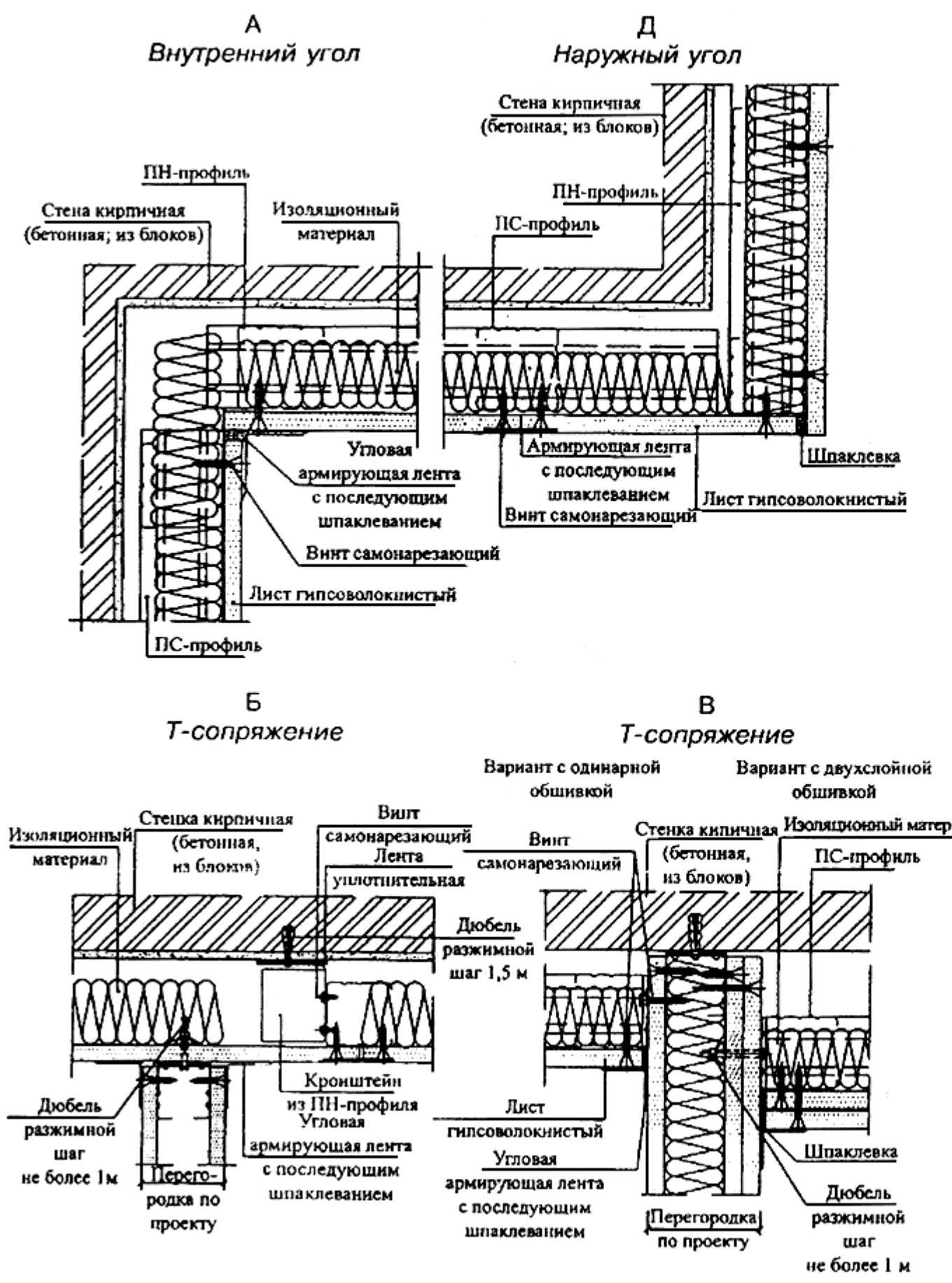
Рисунок 8 - Горизонтальный и вертикальный разрезы, узлы примыканий, внутренние и внешние углы облицовки с одинарной обшивкой гипсоволокнистыми листами по
