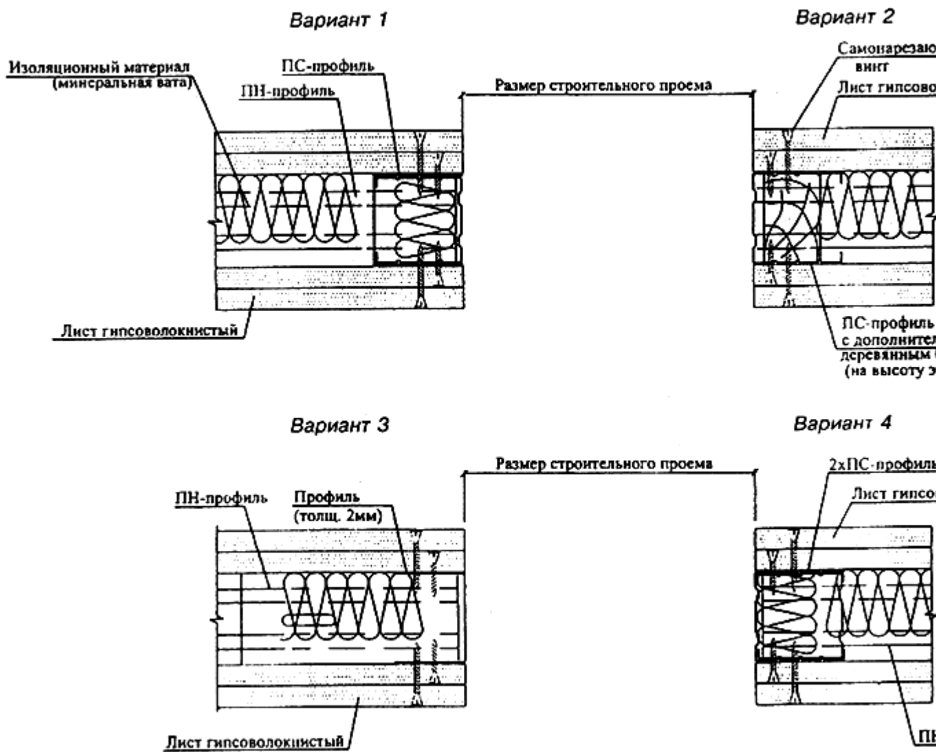
Рисунок 4 - Температурные швы и варианты дверных проемов в перегородках 5.2.2.11 В местах сопряжения перегородок с коммуникационными трассами следует предусматривать установку между стойками каркаса обрамляющих элементов из профилей ПН и ПС с закреплением их к стойкам (рисунок 5).
