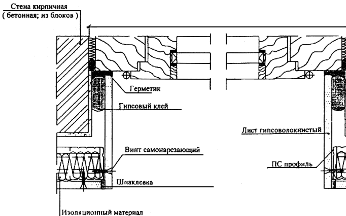
Рисунок 9 - Температурные швы, оконный или дверной проем при облицовке стен
