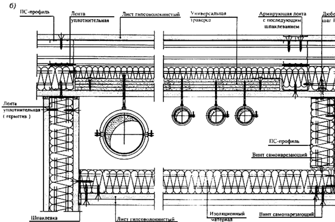
Рисунок 11 - Конструктивные решения ограждения коммуникационных шахт у несущей стены (а) и у перегородки (б)
