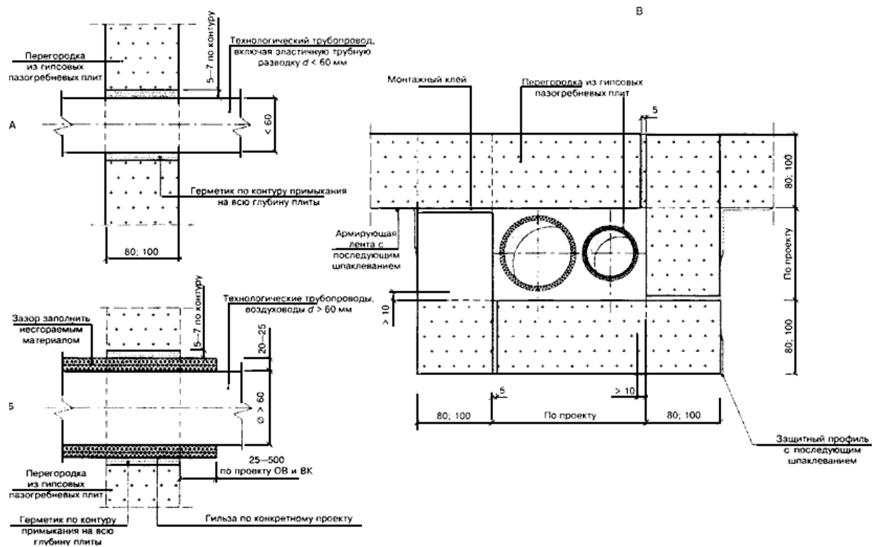
Рисунок 8 - Конструкции узлов пропуска трубопроводов диаметром до 60 мм (А) и более (Б) через перегородку и через шахту (В)
