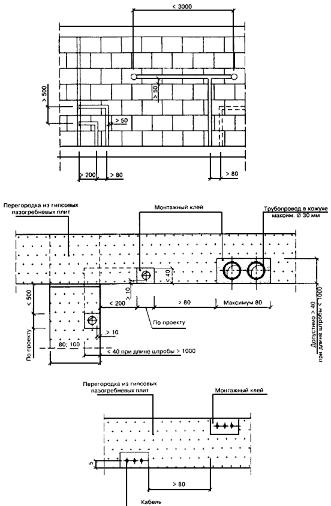
Рисунок 15 - Принципиальные схемы размещения трубопроводов, электрической и слаботочной проводки в перегородках из гипсовых пазогребневых плит 6.2.2 Под розетки, распределительные коробки и выключатели в перегородке или облицовке отверстия высверливаются электродрелью со специальной насадкой.
