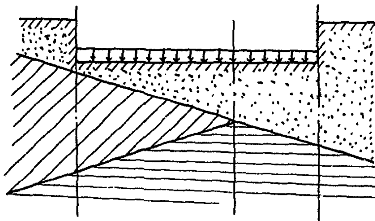
Черт. 1. Геологический разрез неоднородного основания
