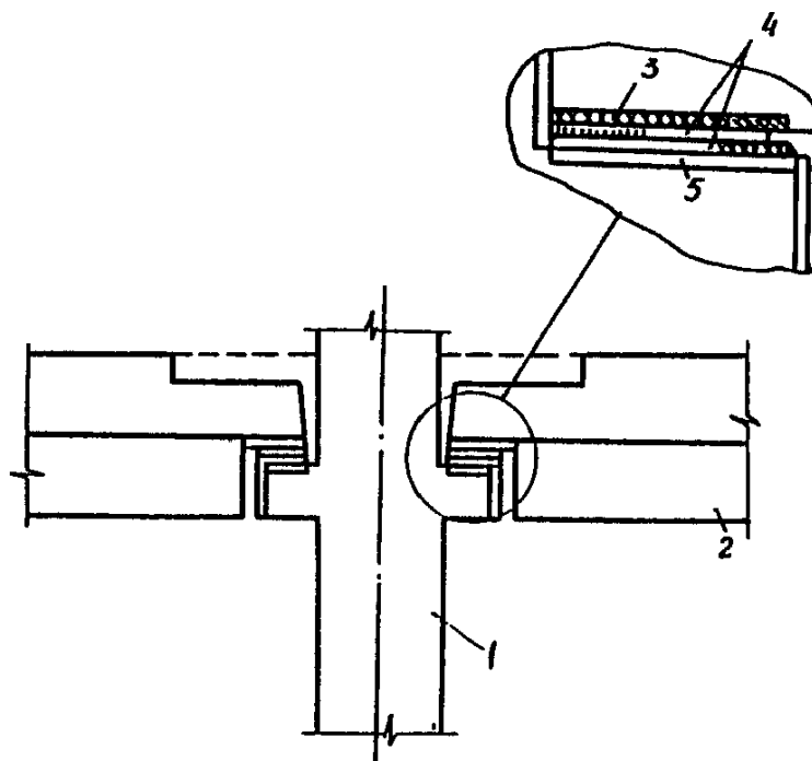
Черт. 2. Конструкция узла сопряжения ригелей с колонной
