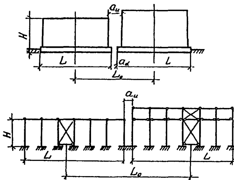
Черт. 3. Схемы для определения размеров деформационного шва между отсеками
