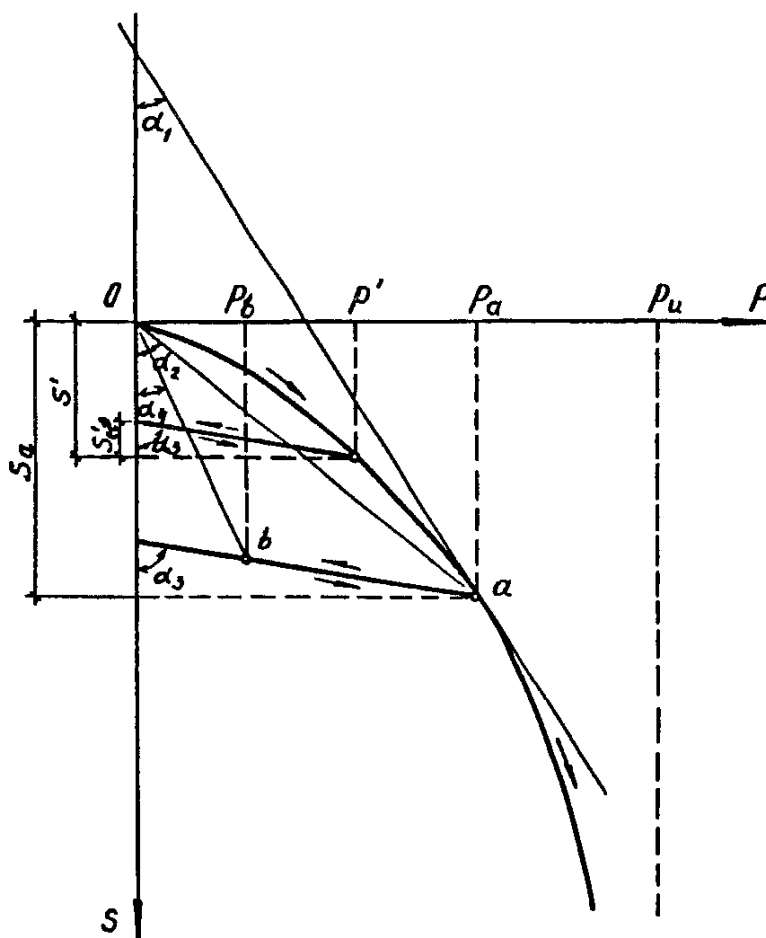
Черт. 2. Расчетная зависимость между осадкой и давлением (нормальным контактным напряжением) для нелинейно-деформируемого основания
