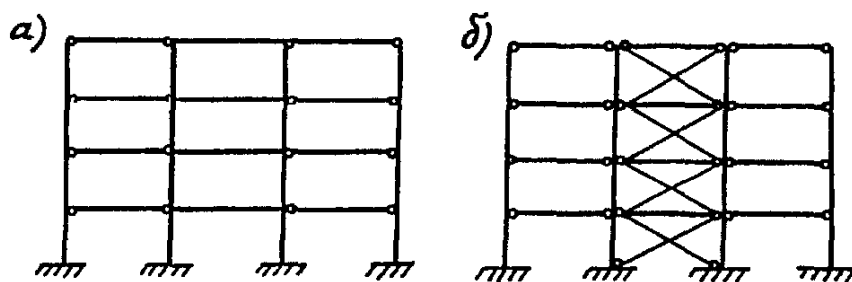
Черт. 1. Схемы рам каркасов многоэтажных зданий
