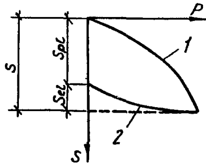
График зависимости осадки от давления при испытаниях грунта штампом
