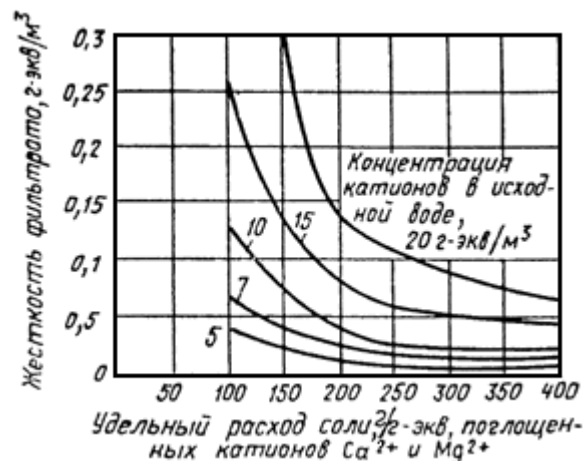
Рис.1. График для определения остаточной жесткости воды, умягченной одноступенчатым натрий-катионированием. Концентрацию регенерационного раствора для фильтров первой ступени следует принимать 5-8%.
