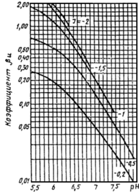
Рис.4. Номограмма для определения коэффициента \beta_{щ} при расчете дозы щелочи
