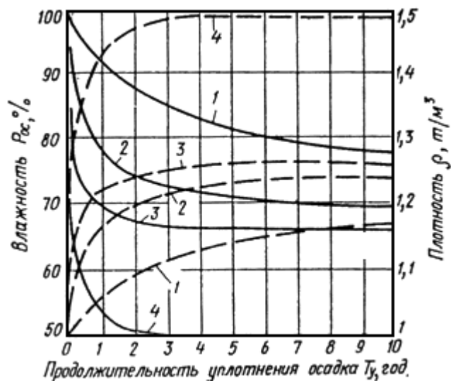
Рис.2. Средние значения влажности и плотности осадка станций обезжелезивания или реагентного умягчения воды при многолетнем уплотнении 1 - реагентное обезжелезивание; 2 - безреагентное обезжелезивание; 3 - реагентное умягчение при магниевой жесткости более 25%; 4 - реагентное умягчение при магниевой жесткости менее 25%
