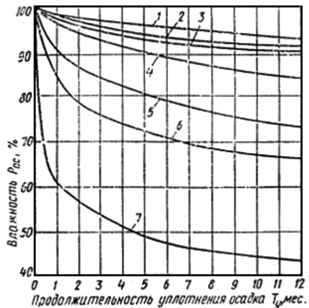
Рис.3. Средние значения влажности осадка станций осветления и обезцвечивания воды при уплотнении до одного года
