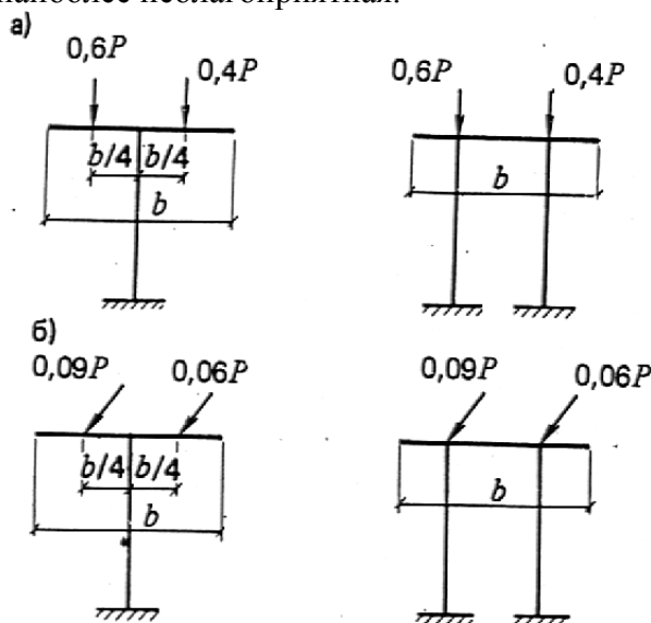
Черт.9. Распределение нагрузки при расчете колонн и фундаментов промежуточных отдельно стоящих опор по поперечному сечению трассы а - схема распределения вертикальной нагрузки; б - то же, горизонтальной нагрузки; P = pb - нормативная вертикальная нагрузка на опору или на соответствующий ярус
