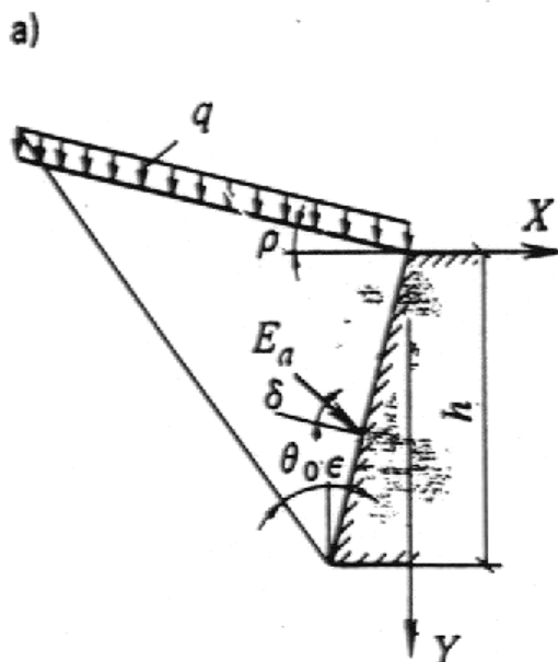
Черт. 1. Схема давления грунта
