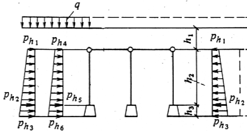
Черт.2. Расчетная схема поперечной рамы подвала
