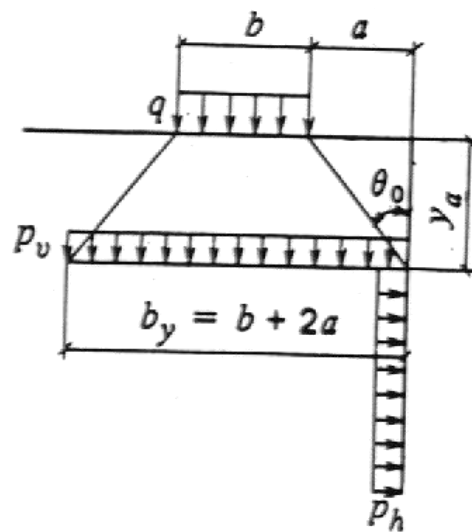
Черт.2. Схема распределения давления от полосовой нагрузки
