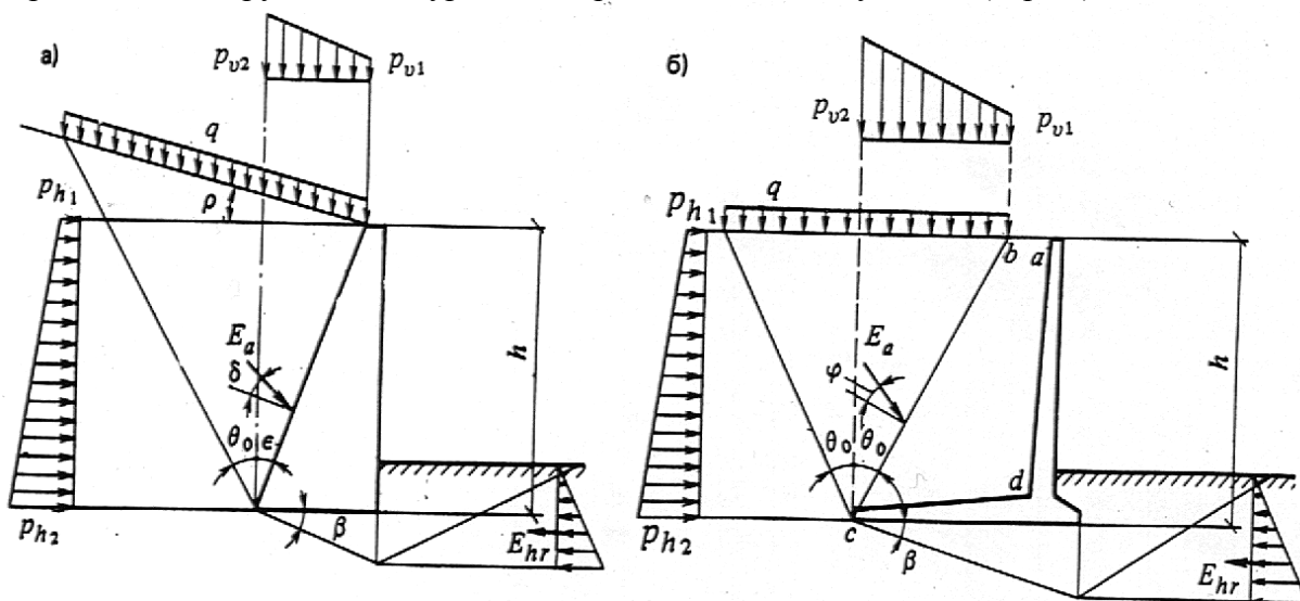
Черт.1. Расчетные схемы подпорных стен а - массивных; б - уголкового профиля
