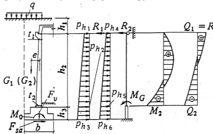
Черт.3. Расчетная схема стены подвала
