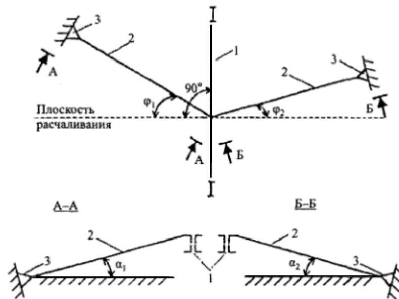
1 - ферма; 2 - расчалка; 3 - якорь
