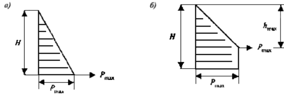
a - гидростатическое давление; б - расчетное давление при уплотнении смеси внутренними вибраторами
