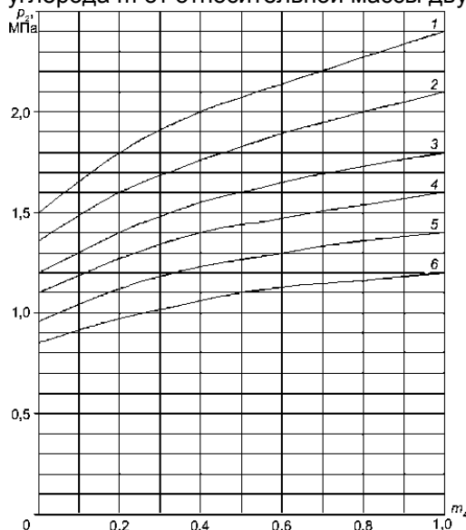
Рисунок Б.1. Зависимость давления p_2 в изотермическом резервуаре в конце выпуска расчетного количества двуокиси углерода m от относительной массы двуокиси углерода m_4
