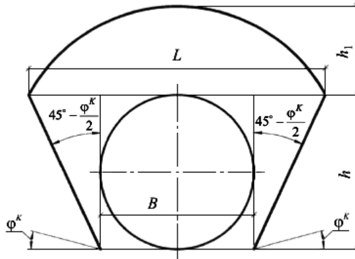
Рисунок 1 - Схема для расчета высоты свода обрушения
