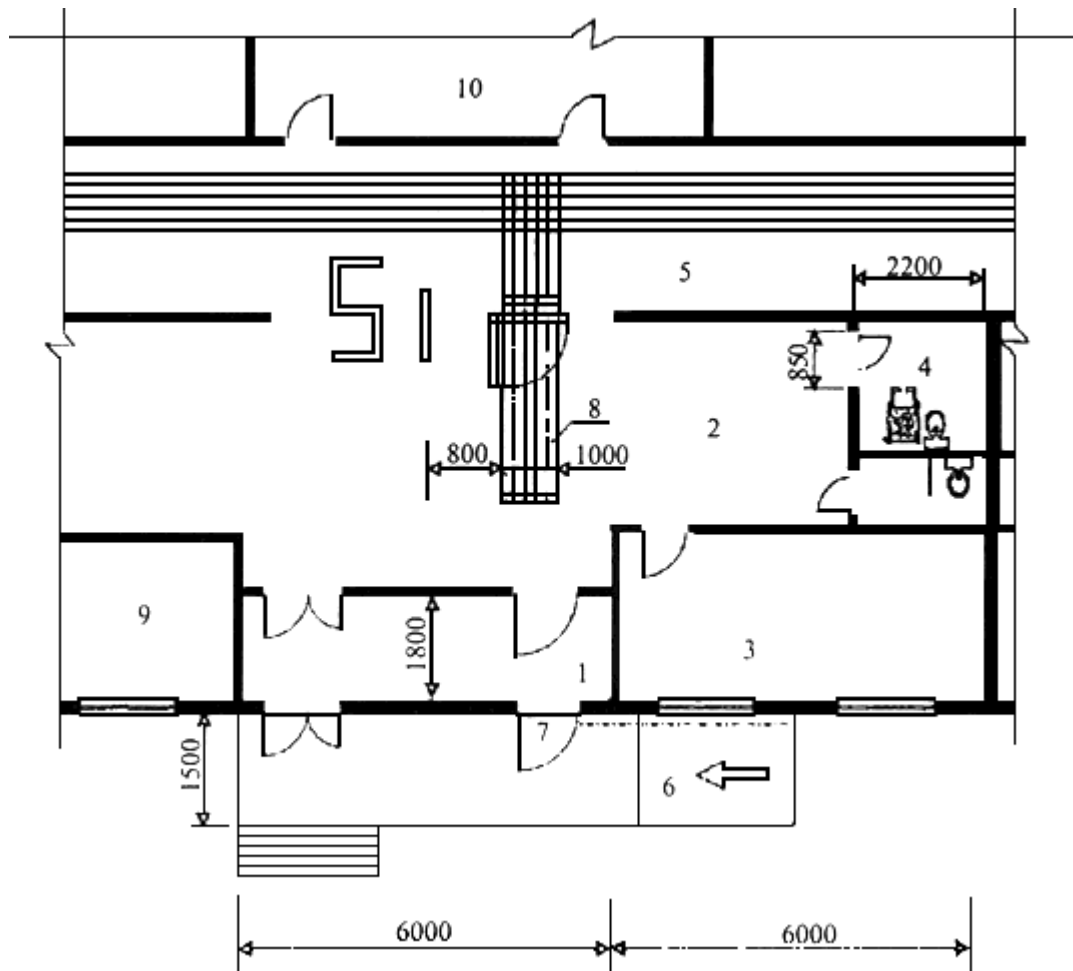
Рисунок В.1 - Рассредоточенное размещение личного транспорта инвалидов
